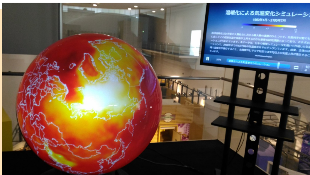
「触れる地球」の温暖化シミュレーション
